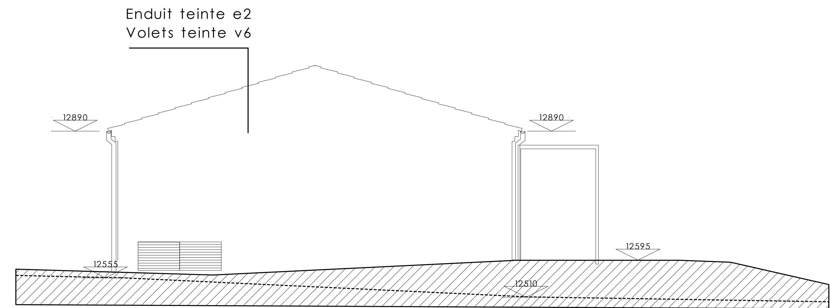
FACADE OUEST VILLA 18
