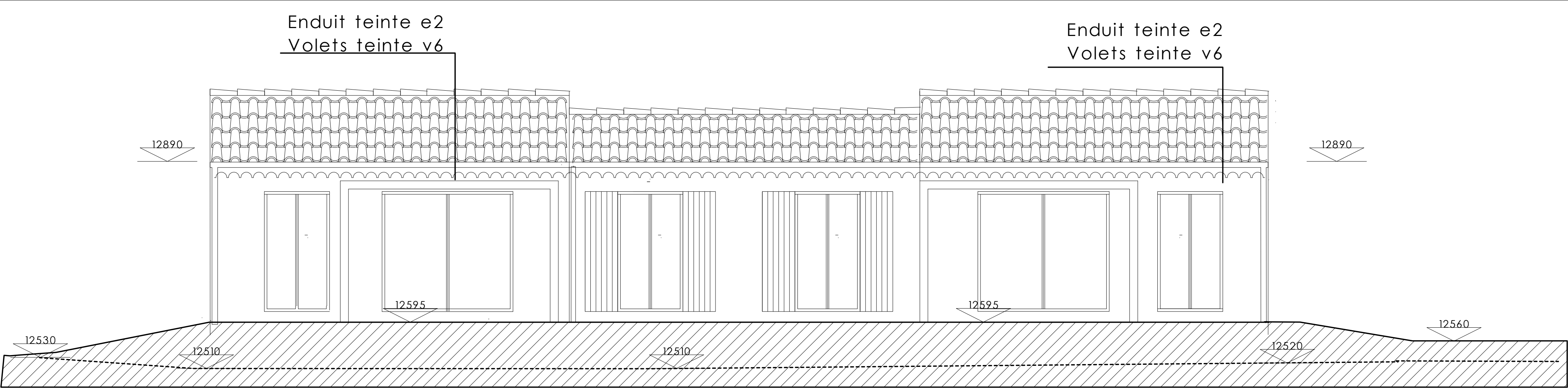
villa 18 FACADES SUD VILLAS 17 ET 18 villa 17
