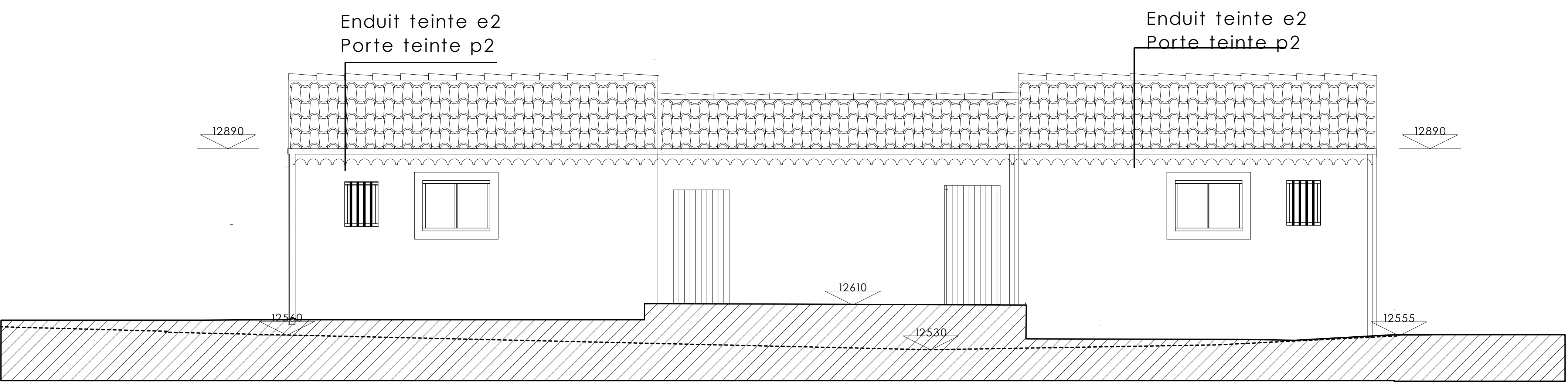
villa 17 FACADES NORD VILLAS 17 ET 18 villa 18
